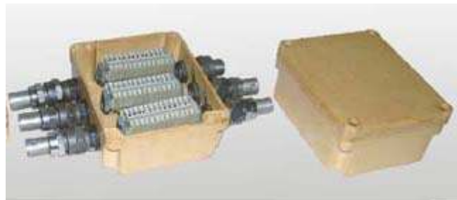
КП-24-00-(3)-42-00-БЗГЗ-G1/2-05-0X-12 Комплект КП-24 (корпус + крышка)
