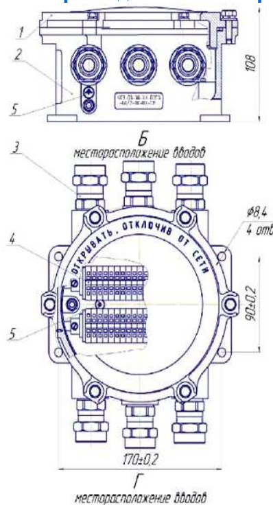
1-крышка, 2-корпус, 3-ввод кабельный, 4-клеммник, 5-знак заземления, 6-зажим заземления
